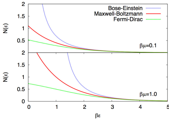
Figura 8.2: Comparação entre as distribuições de Maxwell-Boltzmann (clássica), Bose-Einstein (bósons) e Fermi-Dirac (férmions). Para \beta\epsilon \rightarrow \infty , as três distribuições coincidem. Para \beta\epsilon \rightarrow 0 , bosons tendem a se aglomerar no estado fundamental, enquanto fermions devem respeitar o princípio de Exclusão.
