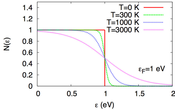
Figura 8.1: Distribuição de Fermi-Dirac para diferentes temperaturas. A energia de Fermi neste caso é \epsilon_F = 1\text{ eV} . No zero absoluto, todos os estados com \epsilon < \epsilon_F estão ocupados, enquanto os estados \epsilon > \epsilon_F estão vazios.
