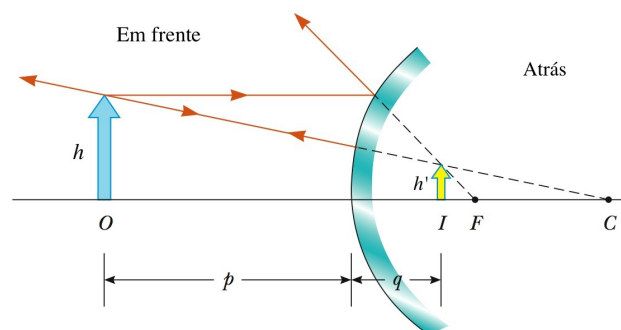
Figura B.6: Espelho Convexo. Situação simétrica a um espelho côncavo em que p < f , invertendo o objeto O e imagem I . (Serway)
