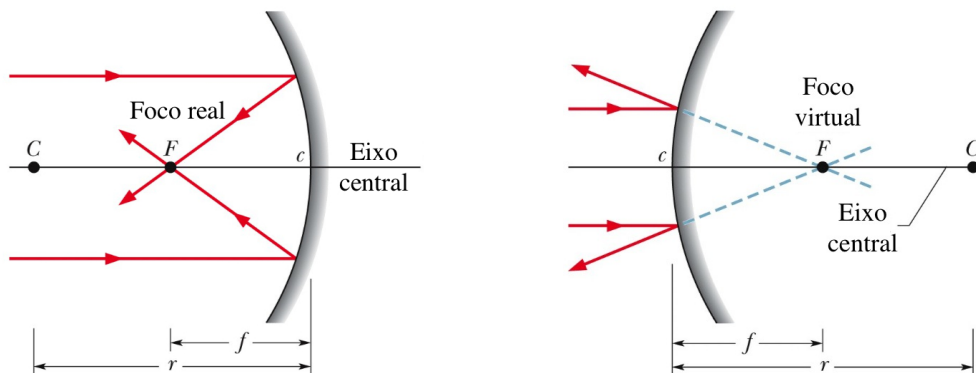
Figura B.4: Foco real (espelho côncavo) e virtual (espelho convexo), definido como o ponto para onde raios incidentes paralelos convergem (foco real) ou de onde os raios paralelos parecem divergir após a reflexão. Para espelhos esféricos f = R/2 . (Halliday)
