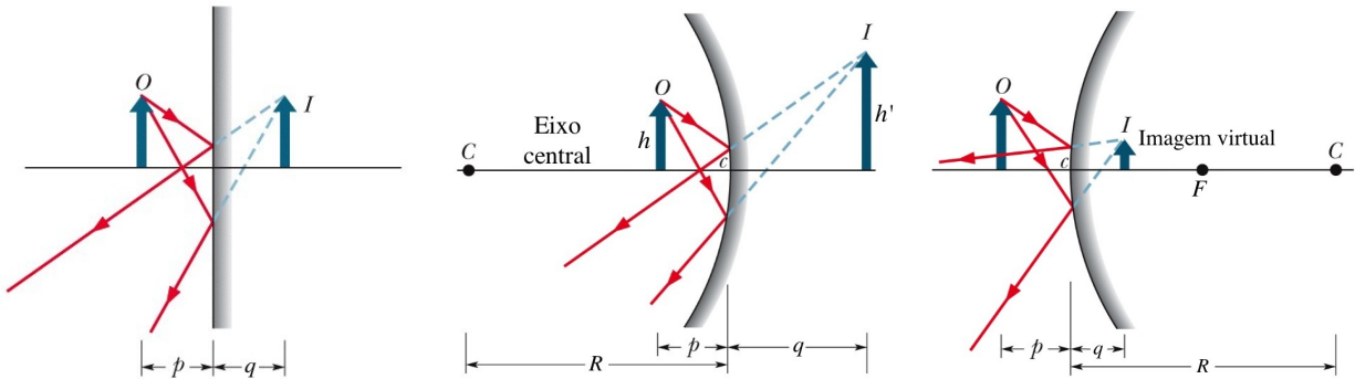
Figura B.3: Espelhos Esféricos. Um espelho plano pode ser deformado, tornando-se um espelho côncavo ou um espelho convexo. As distâncias e alturas das imagem não mais são iguais às do objeto. (Halliday)
