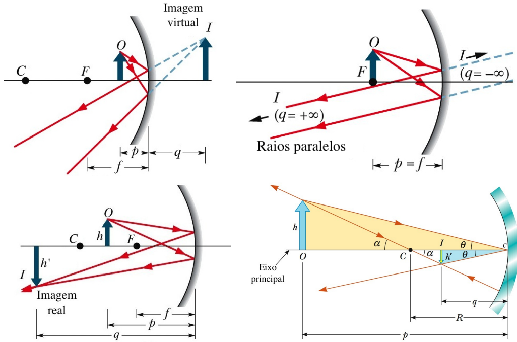
Figura B.5: Espelho Esférico Côncavo. A natureza, posição e altura da imagem dependem da posição do objeto relativa ao foco F e ao centro C . (Halliday, Serway)
