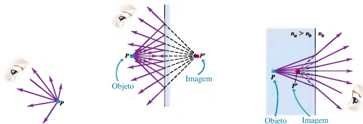
Figura B.1: Podemos ver um objeto olhando para ele ou para a sua imagem refletida/refratada. (Young)
