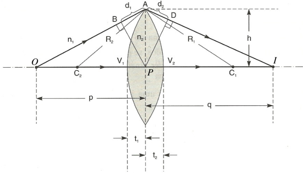
Figura B.11: Lente Biconvexa e o Princípio de Fermat: t_{OAI} = t_{OPI} . (Nussensveig)
