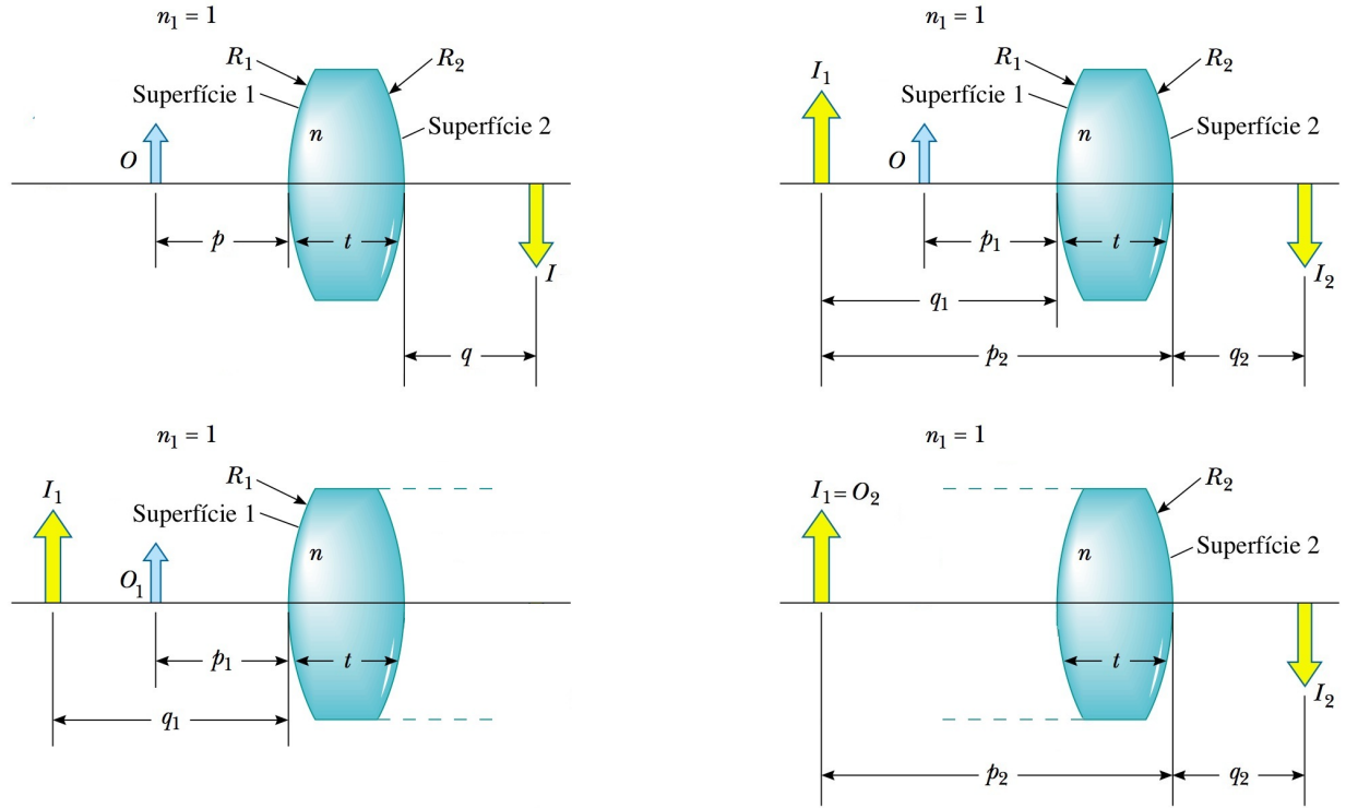
Figura B.10: Lente biconvexa delgada ( t \approx 0 ) vista como duas superfícies. (Serway)
