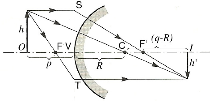
Figura B.8: Refração de um objeto extenso em uma superfície esférica convexa. (Nussenzweig)
