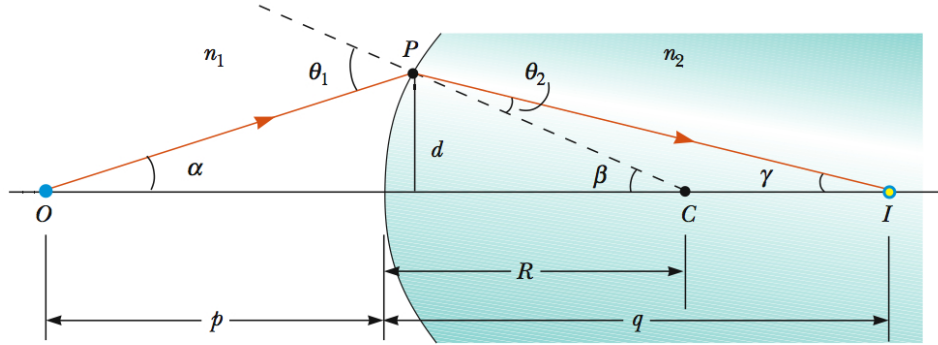
Figura B.7: Refração de um raio de luz em uma superfície esférica convexa com n_2 > n_1 . (Serway)
