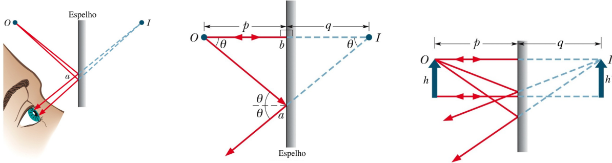
Figura B.2: Espelho Plano. Como consequência da lei da reflexão, a distância do objeto ao espelho é igual à distância da imagem ao espelho. (Halliday)
